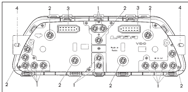
Рис. 50. Комбинация приборов
