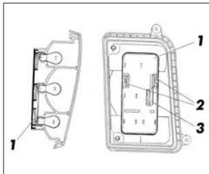
Рис. 47. Задний фонарь
