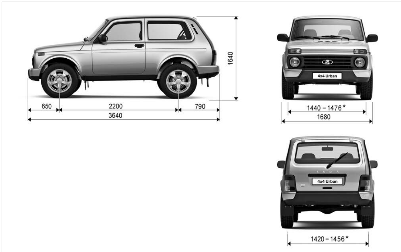
Рис. 57. Габаритные размеры автомобиля LADA 4x4 Urban 3 дв.
