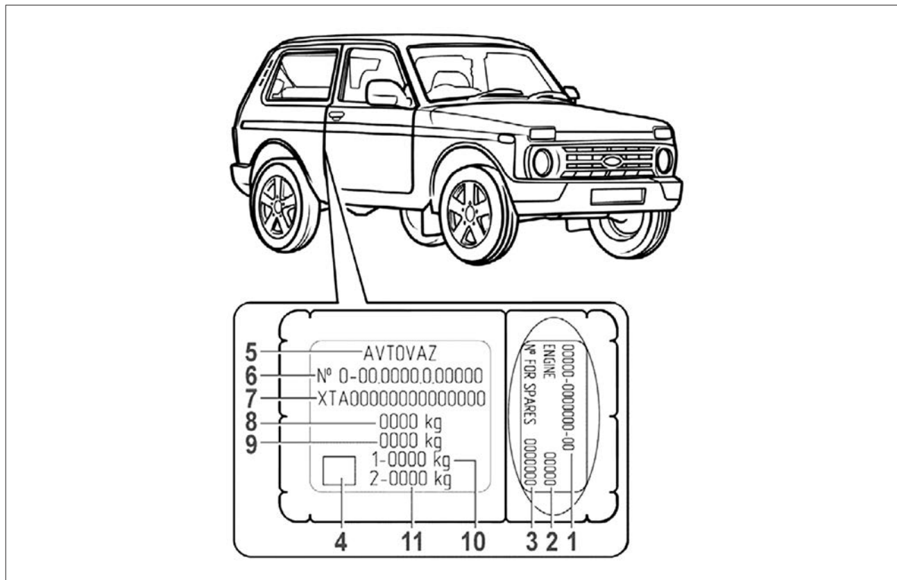
Рис. 59. Паспортные данные. Место установки таблички: 21214 – панель боковины правой; 2131 – панель боковины средней правой
