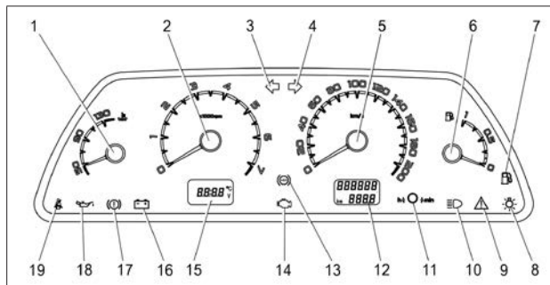
Рис. 13. Комбинация приборов
