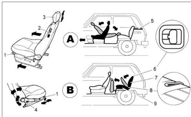
Рис. 8. Сиденья
