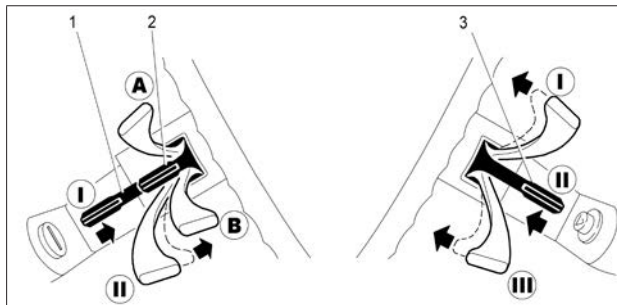
Рис. 14. Подрулевые переключатели
